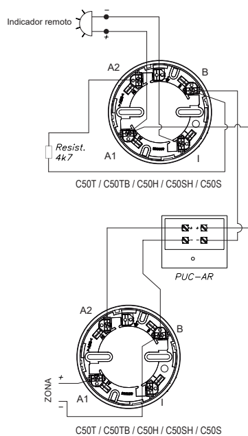
Esquema de conexionado
