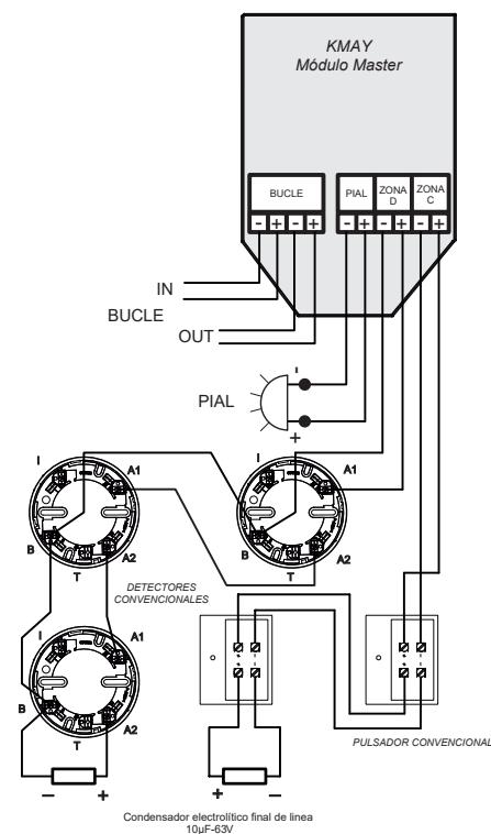
Esquema de conexionado
